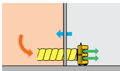
Luchtreiniging op basis van onderdruk, waar Dryfast de voorkeur aan geeft.
