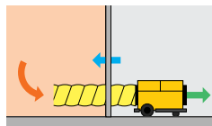
Onderdrukhandhaving buiten de ruimte via een luchtslang.
